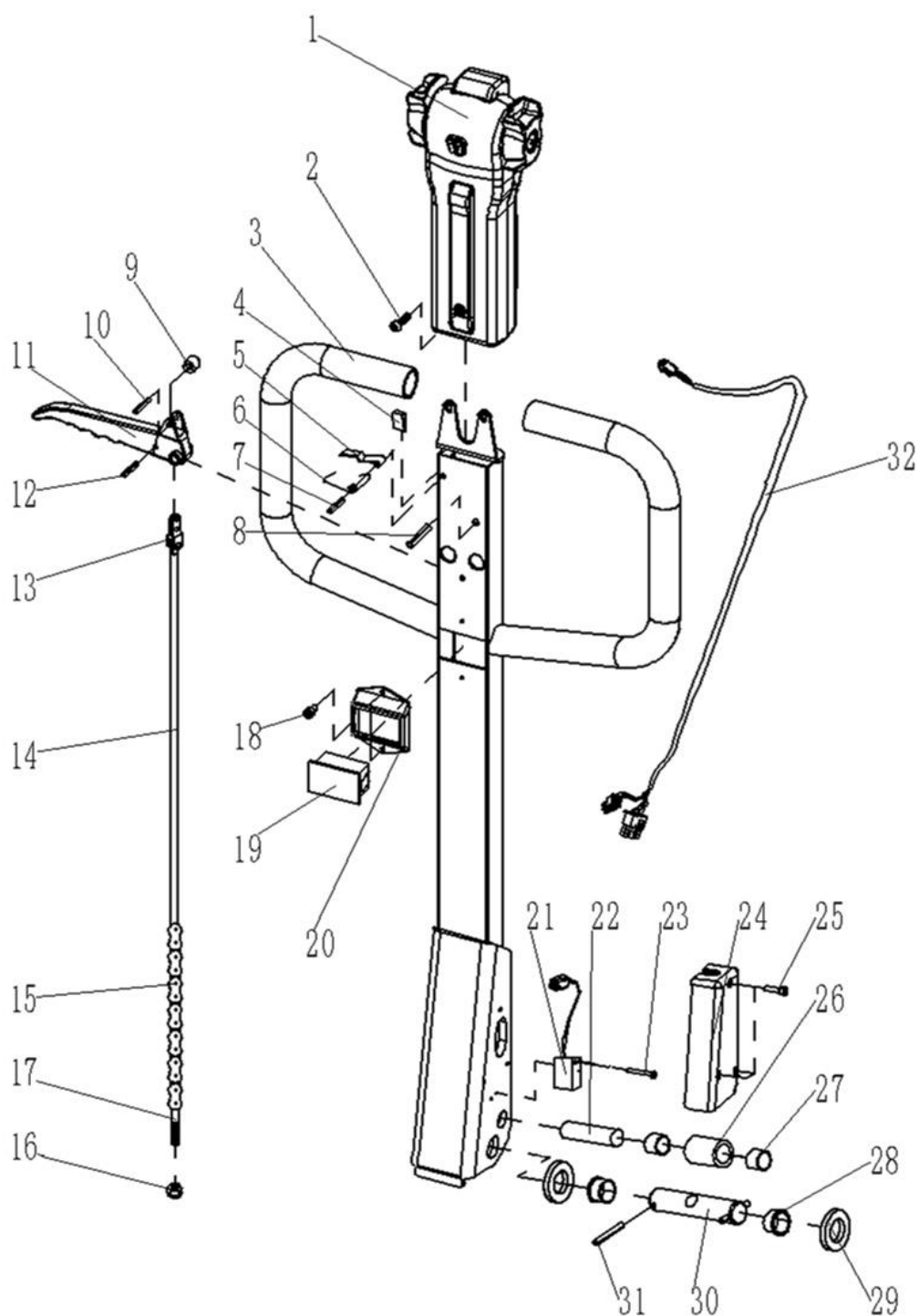
Fig.10 Handle bar (SPTE15X)
