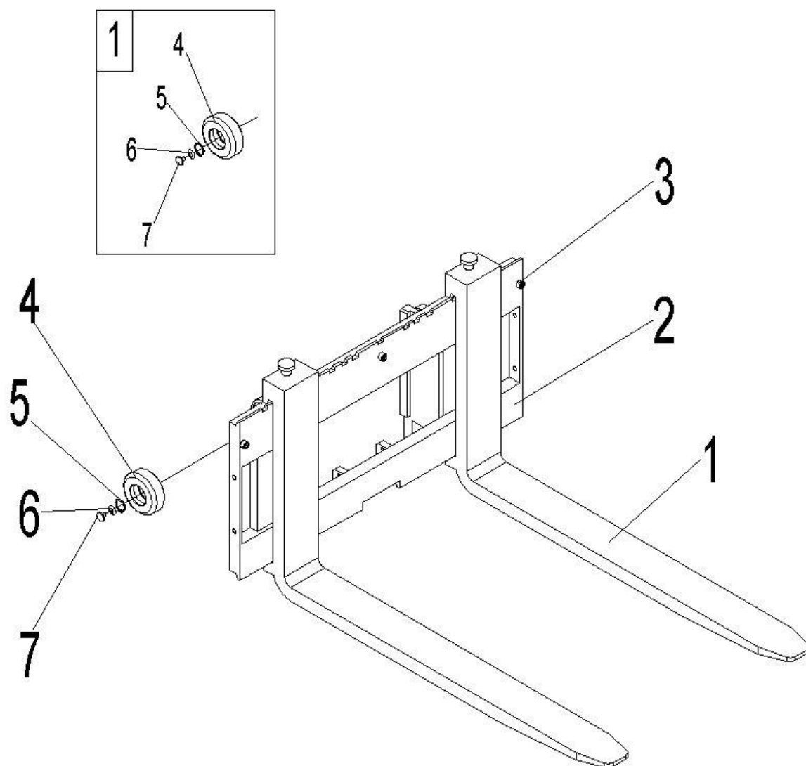
Fig. 4 Fork
