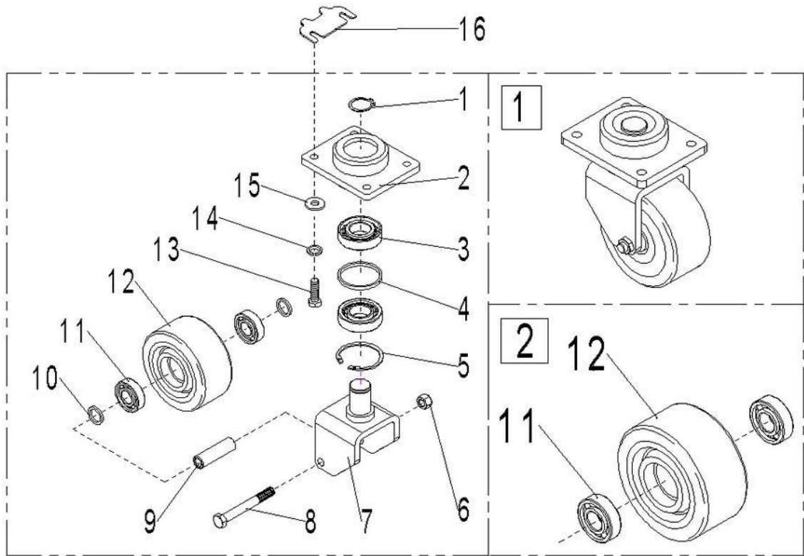
Fig. 6 Castor
