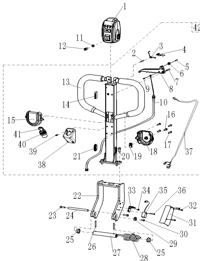
Fig. 7 Handle Bar
